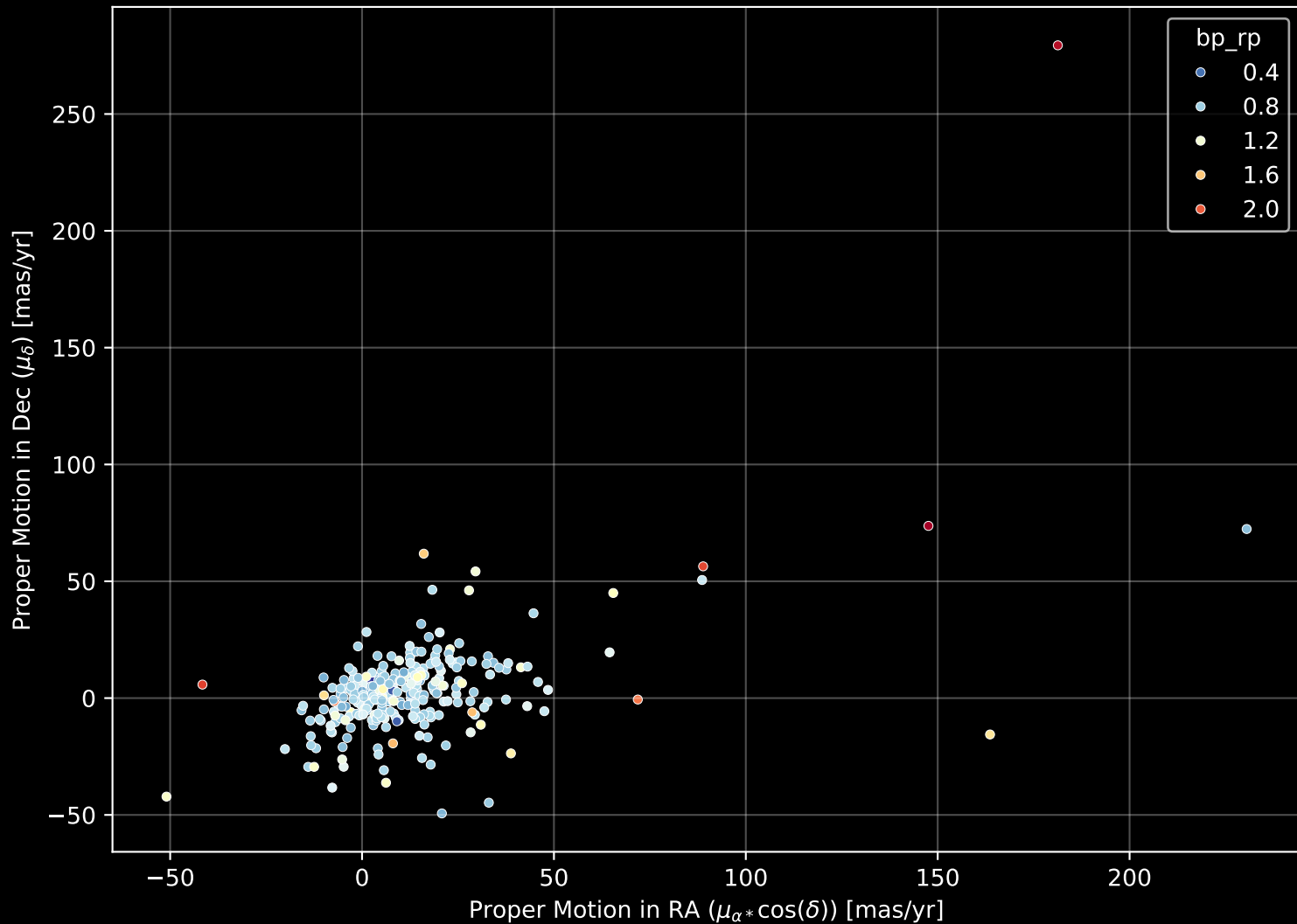
GALAH DR4 Field: [6958] Proper Motion Diagram (n= 289)
