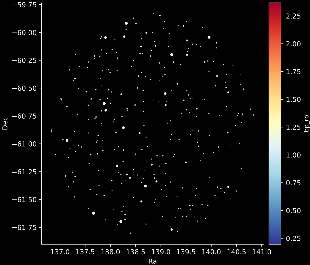
GALAH DR4 Field: [6958] Stars: 289
