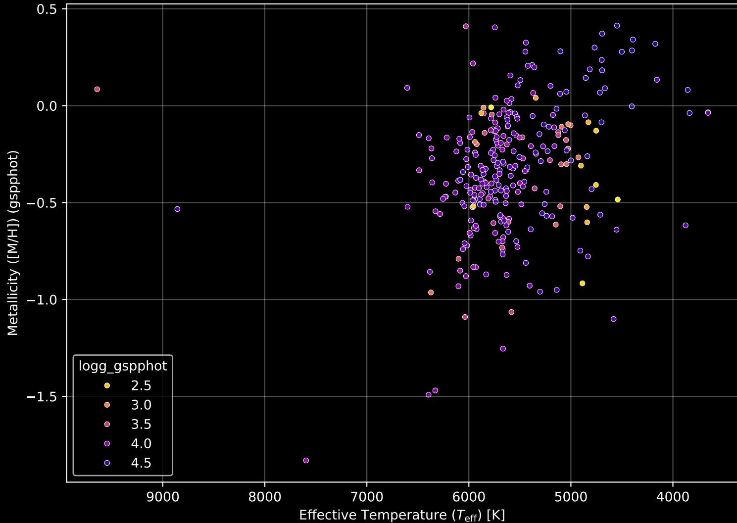
GALAH DR4 Field: [6958] Stellar Population Parameters (n= 289)
