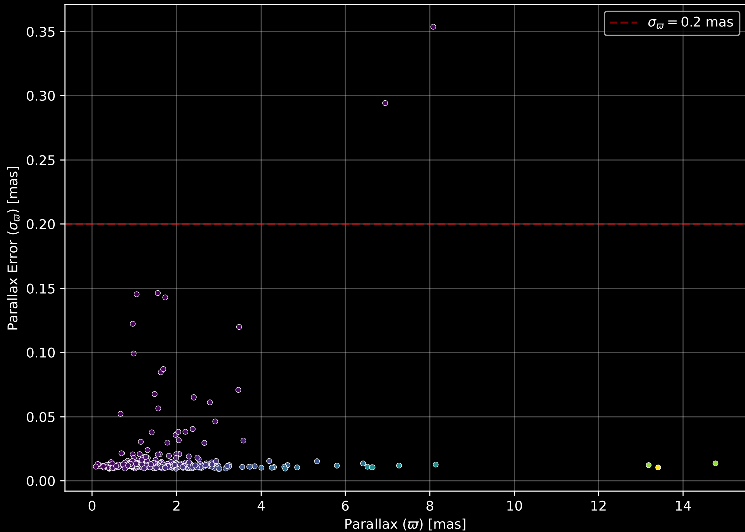
GALAH DR4 Field: [6958] Parallax Quality (n= 289)
