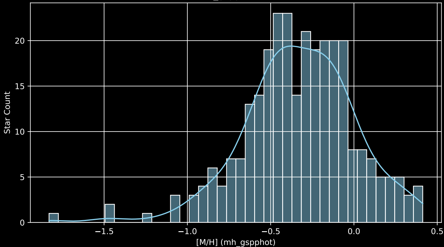
GALAH DR4 Field: [6958] [M/H] (mh_gspphot) (n= 289)
